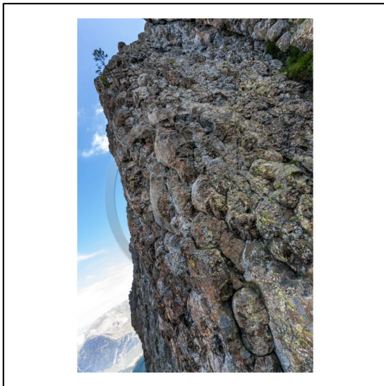
Hauts-Alpes (05), Montgenèvre, Le Chenaillet, Le massif du Chenaillet est le massif des Alpes où les ophiolites sont très bien conservées où l'on y trouve les plus belles laves en coussins (appelées pillow lavas) océaniques de France et d'Europe. // Hauts-Alpes (05), Montgenevre, The Chanaillet, The massif is Chenaillet the Alps where ophiolites are very well preserved where there are the most beautiful pillow lavas Ocean of France and Europe.
