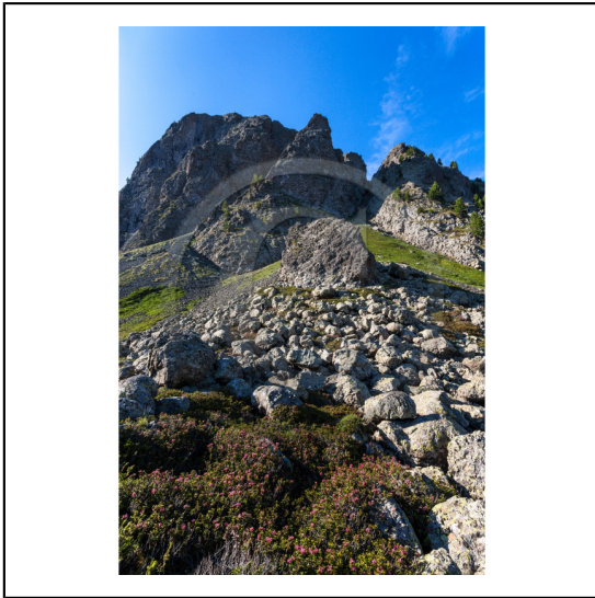
Hautes-Alpes (05), Montgenèvre, Le Chenaillet, Le massif du Chenaillet est le massif des Alpes où les ophiolites sont très bien conservées où l'on y trouve les plus belles laves en coussins (appelées pillow lavas) océaniques de France et d'Europe. // Hautes-Alpes (05), Montgenevre, The Chanaillet, The massif is Chenaillet the Alps where ophiolites are very well preserved where there are the most beautiful pillow lavas Ocean of France and Europe.
